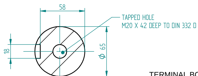
Przekrój A-A 1:2
